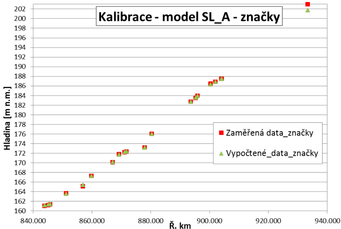
Graf 2 – Kalibrace modelu – úsek Mělník – Týnec, značky
