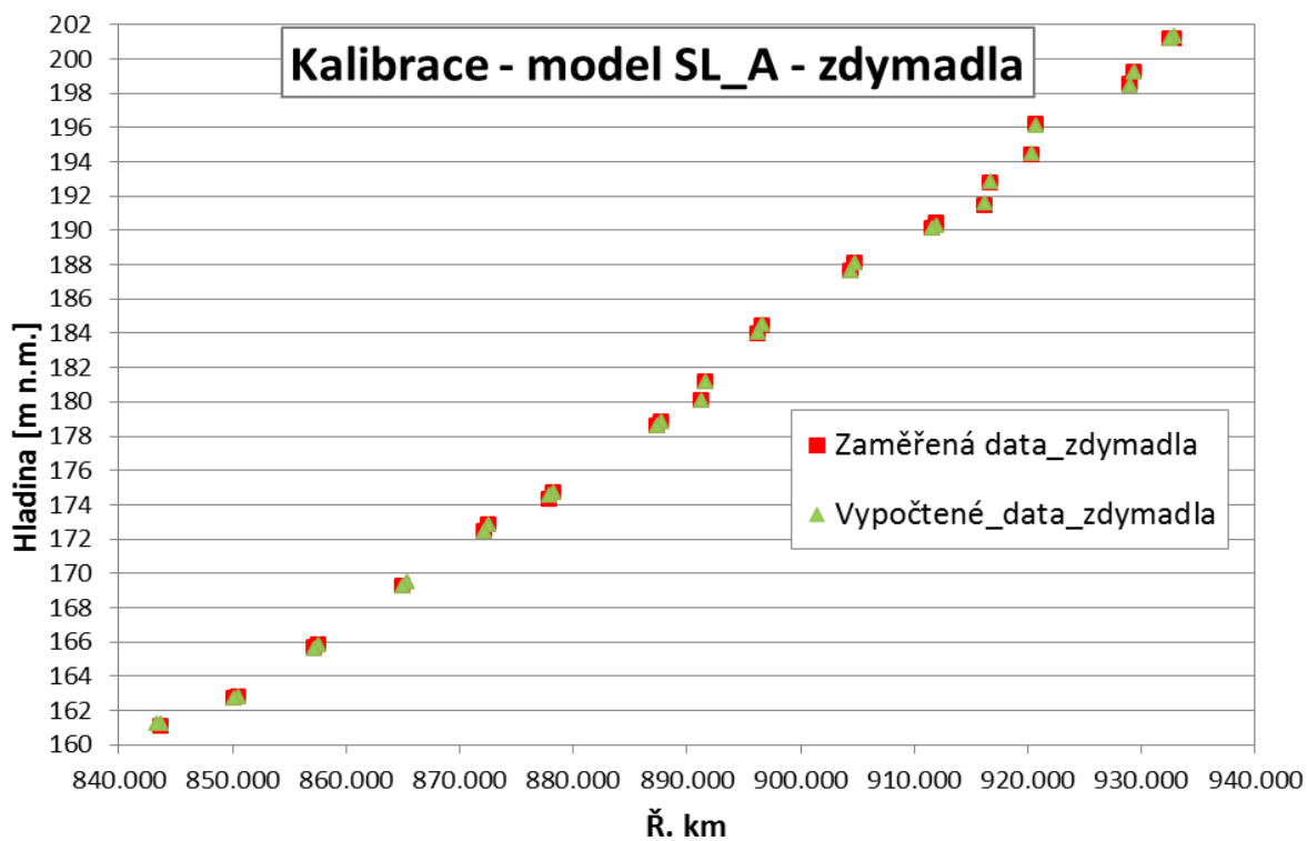
Graf 1 – Kalibrace modelu – úsek Mělník – Týnec, jezy
