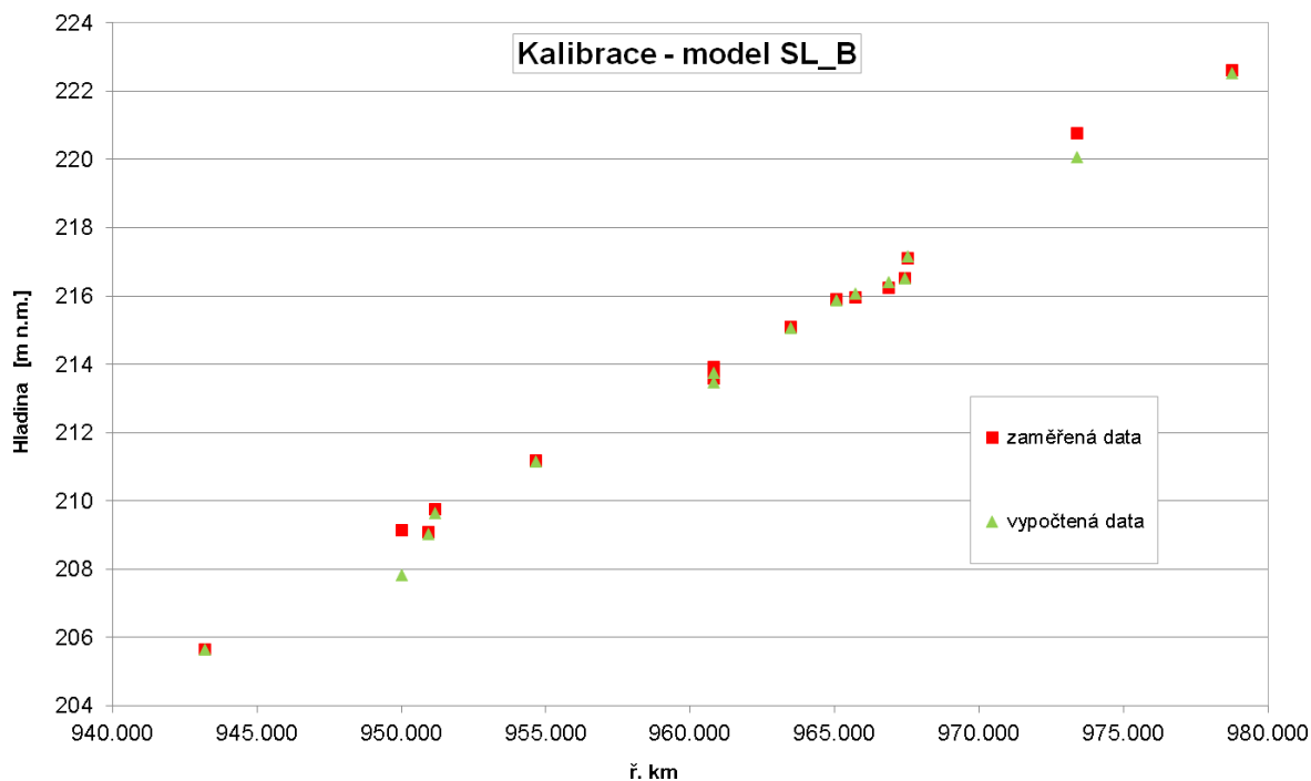
Graf 3 – Kalibrace modelu – úsek Týnec – Opatovice, značky
